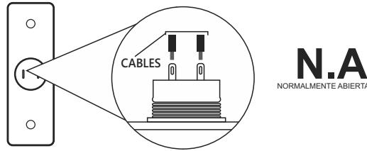
DIAGRAMA DE CABLEADO
