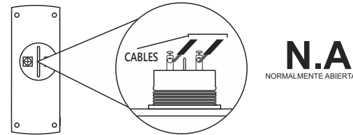
DIAGRAMA DE CABLEADO
